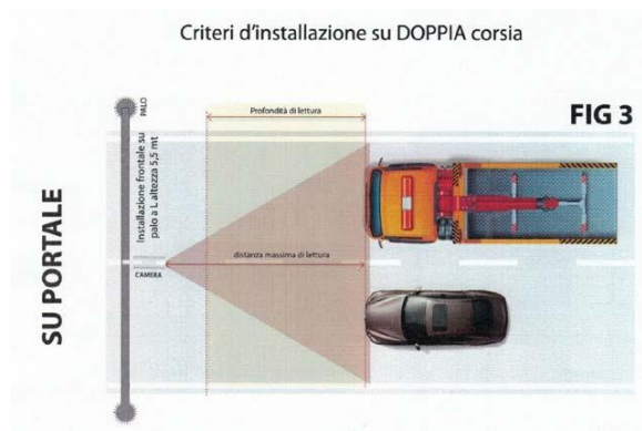
La Fig. 3 mostra le migliori condizioni per una lettura su doppia corsia. Nel caso del senso unico di marcia la situazione migliore la si ha quando la telecamera è installata su portale e puntata verso le targhe frontali in avvicinamento
