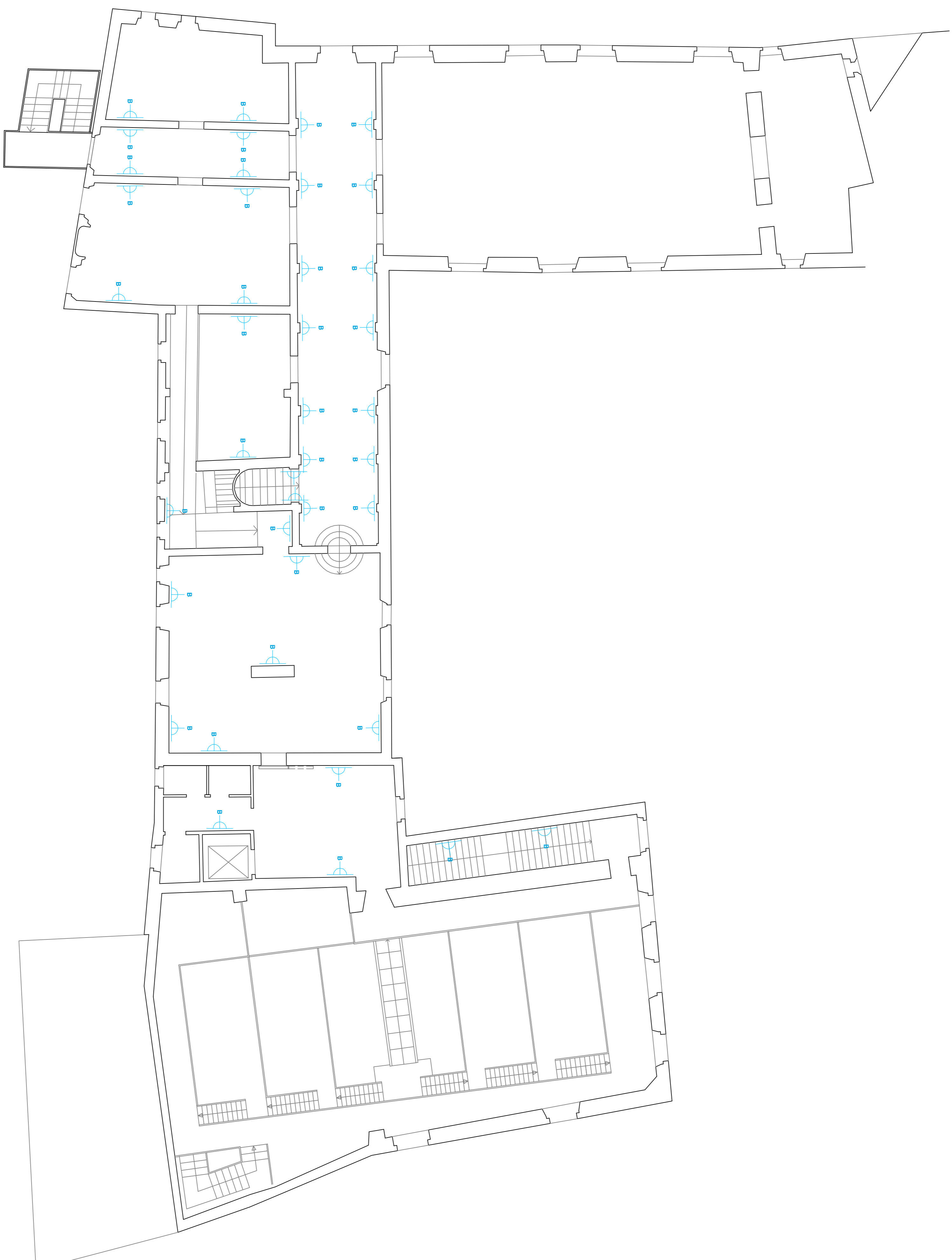
PIANTA PIANO SECONDO
