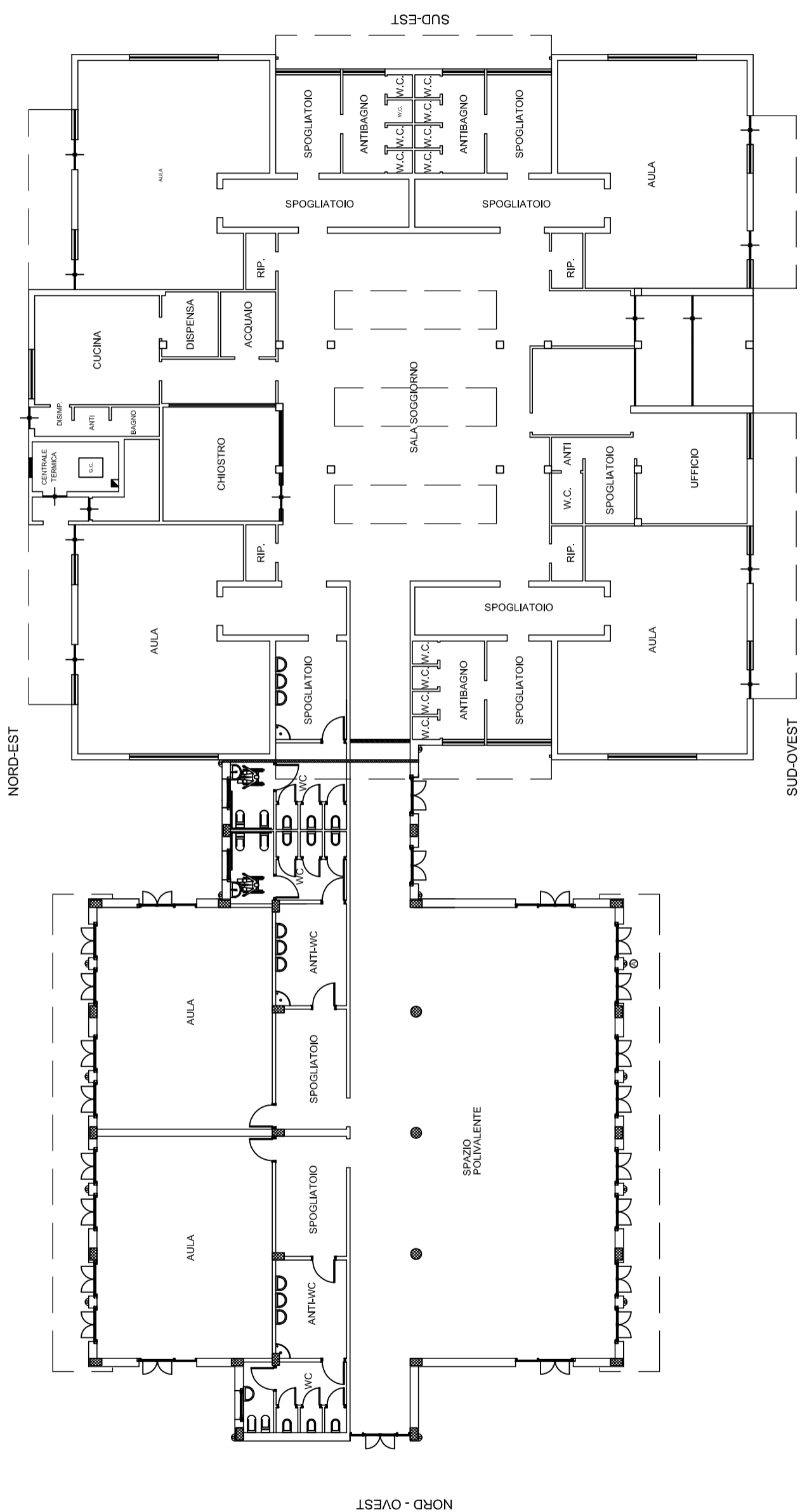
PIANTA Sc.1:200
